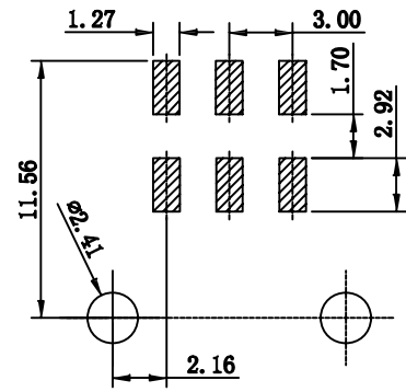
P. C. B. LAYOUT
